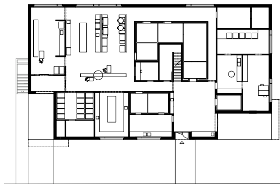
Grundrisse Erdgeschoss und Obergeschoss, rechts: Betriebsschema
